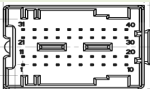
Connector 40 Pin Black (0---953118---1)
