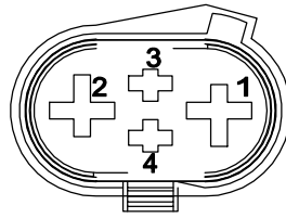
E01 1.5T GDI Cooling fan
