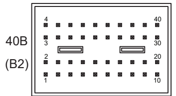
Connector 40 Pin Black (0-953118-1)
