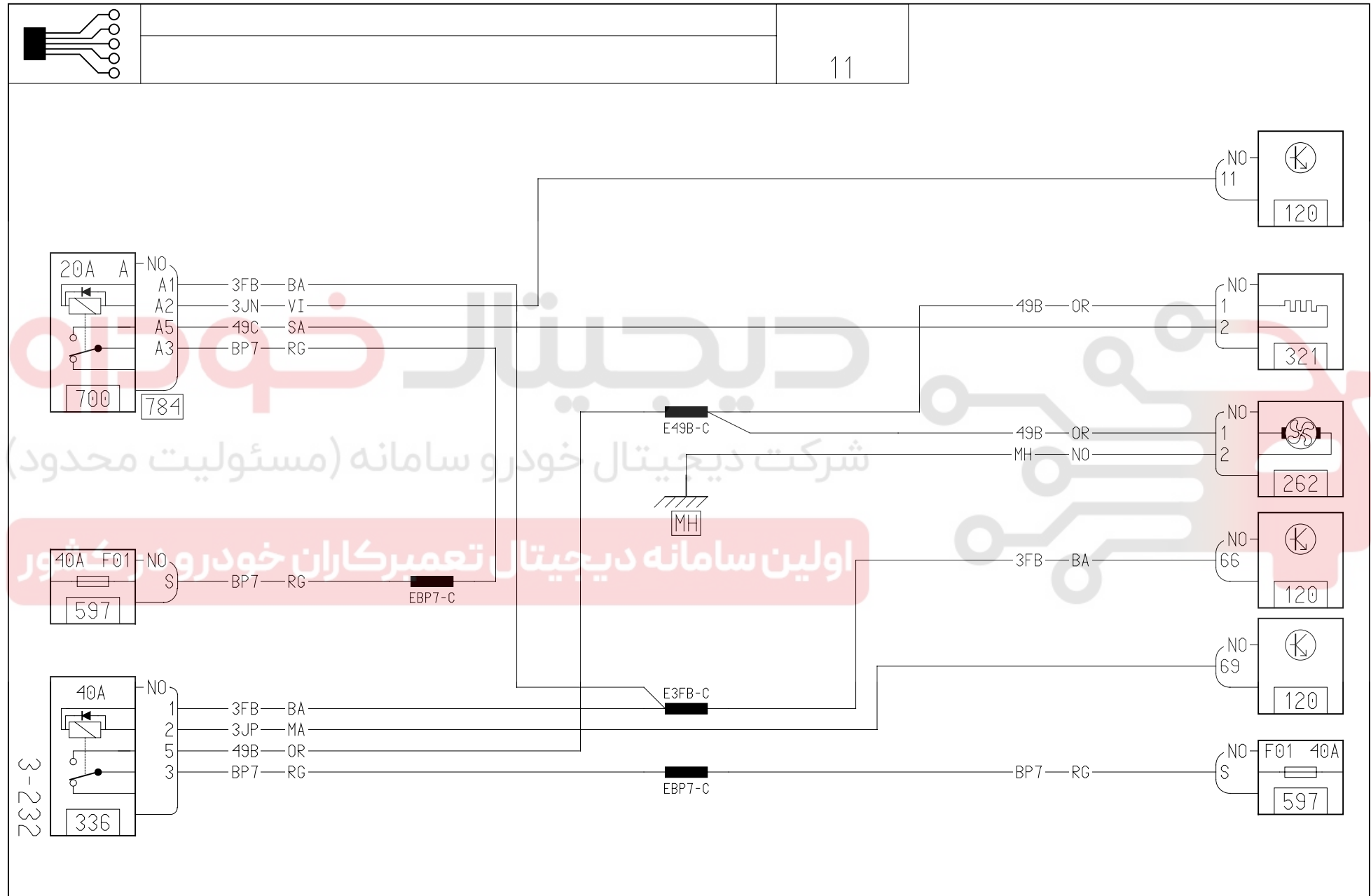
سیستم خنک کننده موتور خودرو دوگانه سوز
