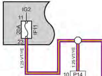
فیوز داشبورد و جعبه رله P01
