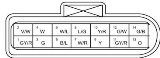
شیر کنترل
