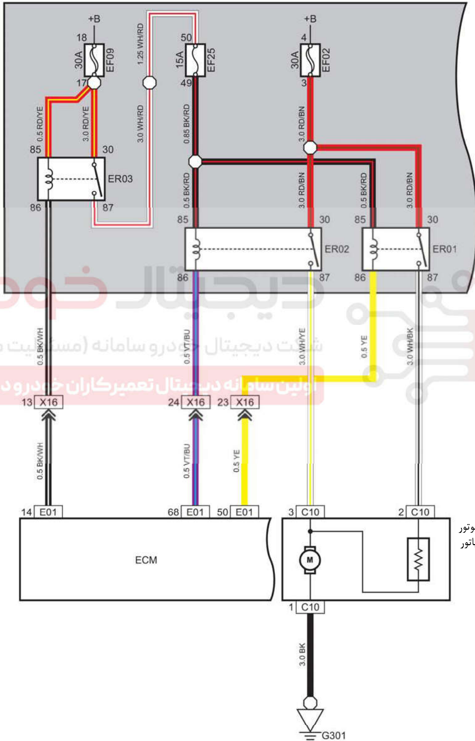
جعبه رله و فیوز محافظه موتور C01
