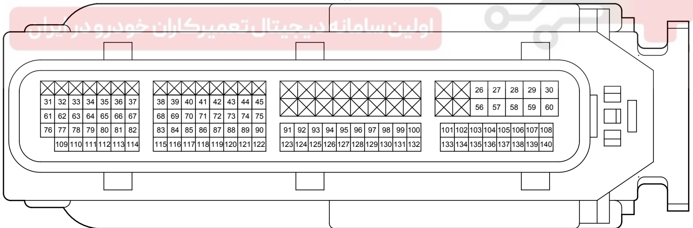
90980-12A38
