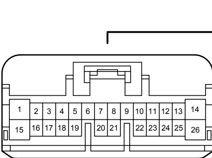
90980-12771
