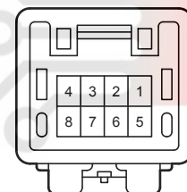
90980-12734
