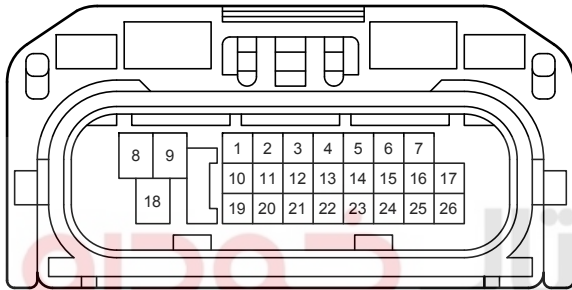
90980-12649
