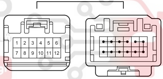
90980-12737
