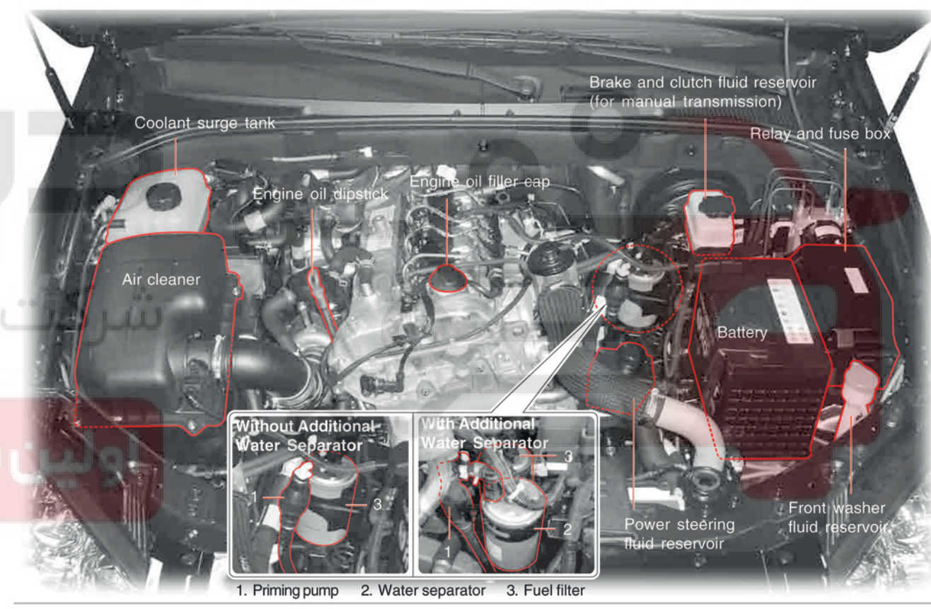
موتور دیزل (D27DT)
